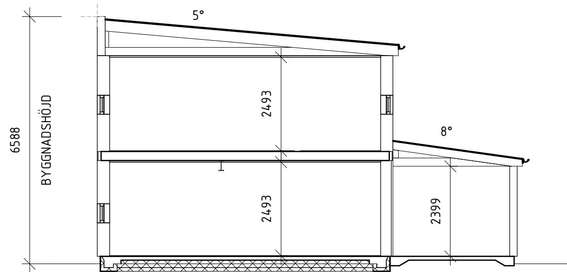
SKÅNETAKFOT SEKTION A-A
